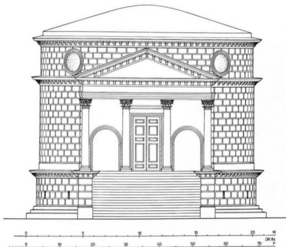
Fig. 5. Ricostruzione del mausoleo dei Gordiani (da Rasch 1993).
