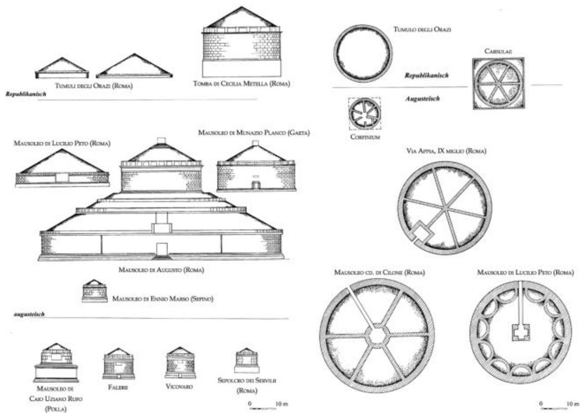
Fig. 4. Tavola comparativa di mausolei a tumulo di età tardo-repubblicana e augustea (rielaborazione dell'A. da Schwarz 2002).
