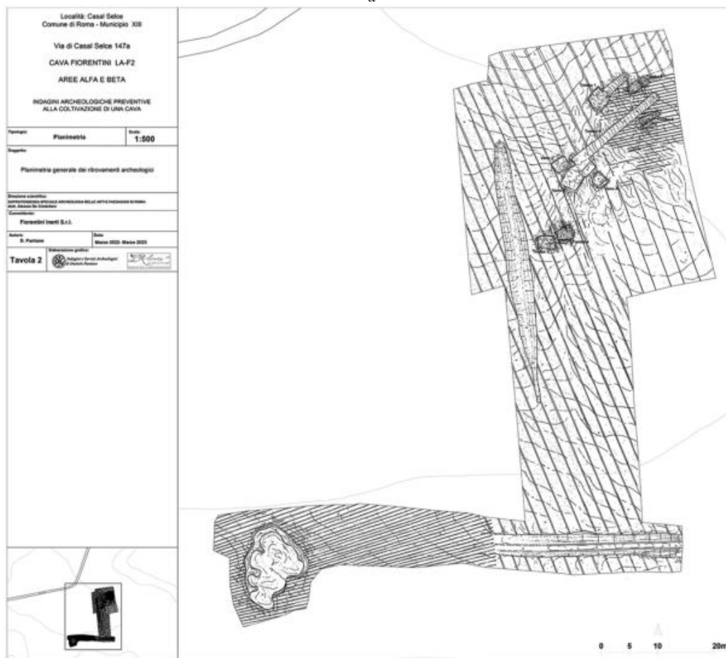
Fig. 1. a) Posizionamento del tumulo di Casal Selce (elab. A. Piergrossi da Google Earth); b) Pianta generale del sito (Kairòs. Servizi per l'Archeologia s.r.l.).
