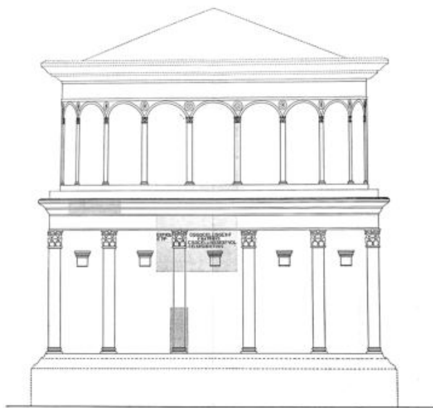
Fig. 3. Proposta di ricostruzione del monumento dei Socelli (da von Sydow 1977, fig. 29).
