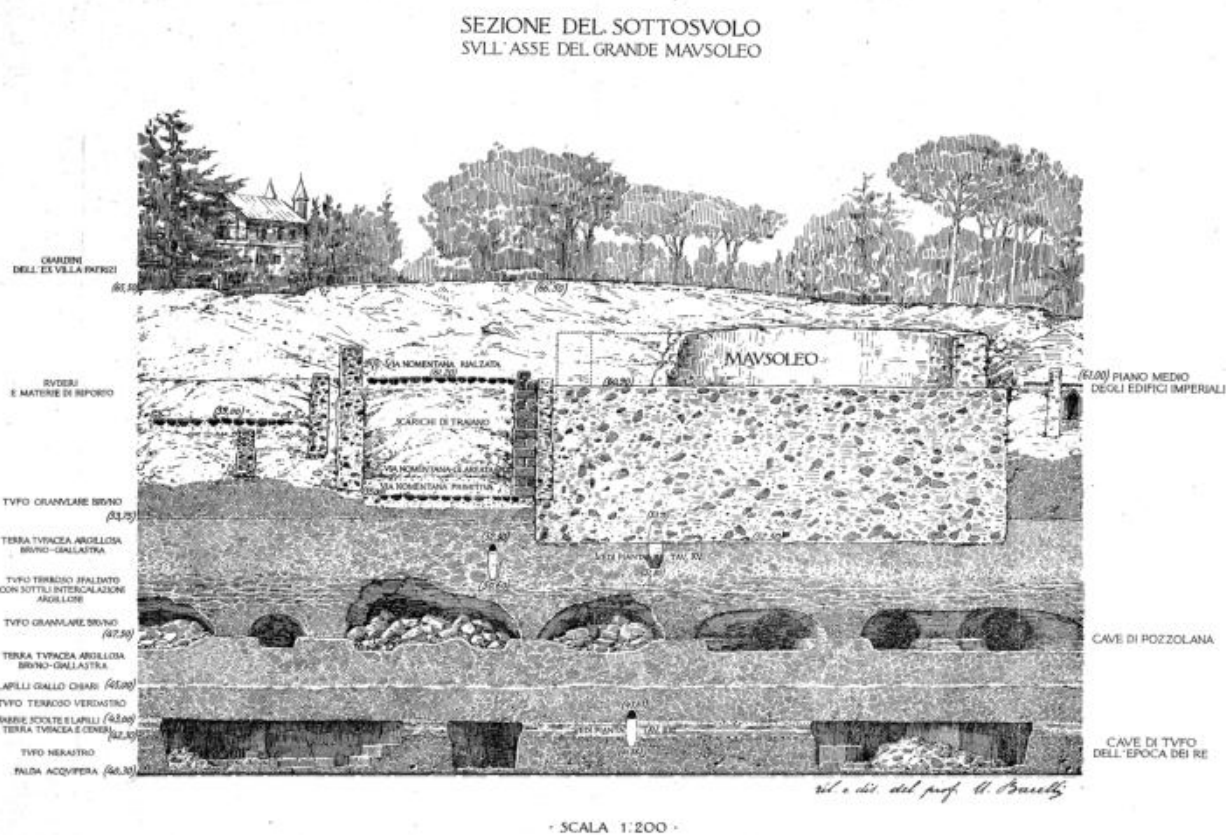
Fig. 3. Sezione del sottosuolo della Villa Patrizi rilevata in corrispondenza del mausoleo (da Lanciani 1918, tav. XVI).
