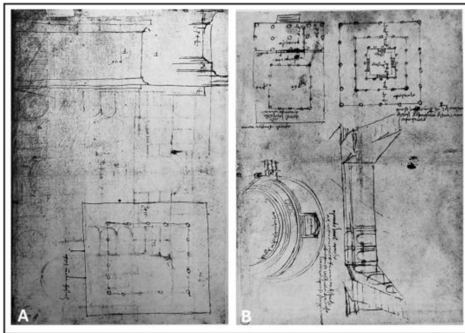
Fig. 5. Francesco di Giorgio Martini, Uffizi 327 (a sinistra) – 328 (a destra) (da Vasori 1980).
