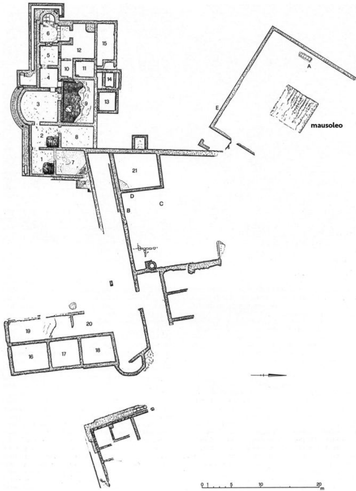
Fig. 8. Guidonia Montecelio (RM), via di Marco Simone. Planimetria della villa con annesso mausoleo (rielaborazione dell'A. da Mari, Moscetti, Rustico 1994-1995, fig. 25).
